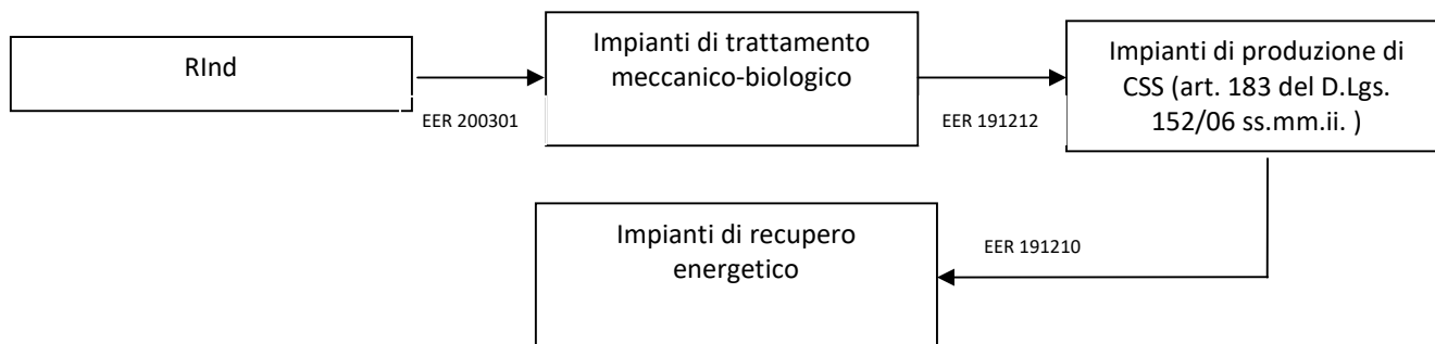
FIGURA 25 - SCHEMA DI FLUSSO GESTIONE RIFIUTI INDIFFERENZIATO – FASE TRANSITORIA
