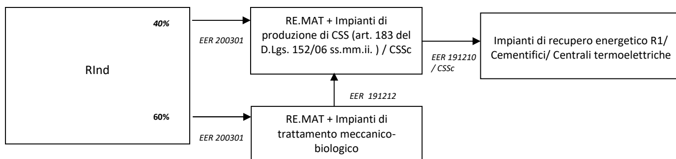
FIGURA 26 - SCHEMA DI FLUSSO GESTIONE RIFIUTI INDIFFERENZIATO – FASE A REGIME
