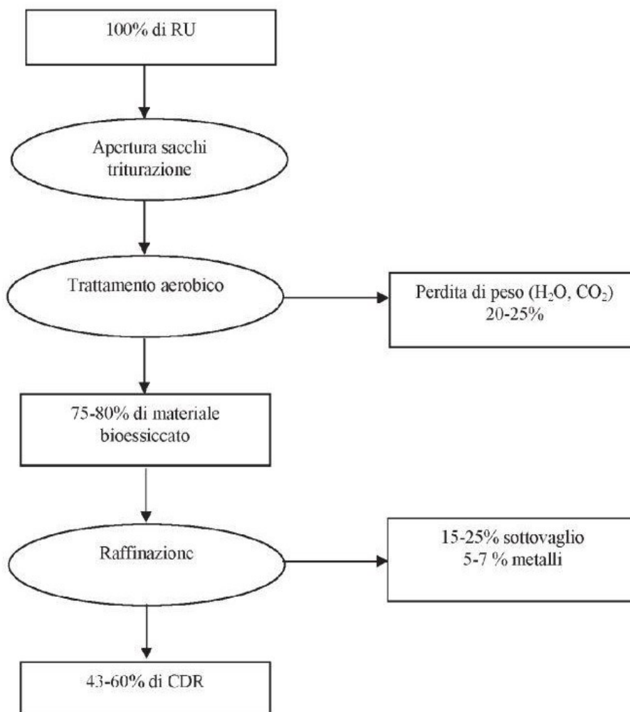
FIGURA 24 – TMB: SCHEMA DI PROCESSO E BILANCIO DI MASSA CON METODO A FLUSSO UNICO
