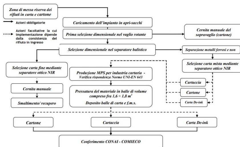
FIGURA 17 –IMPIANTO DI BARLETTA: LAYOUT
