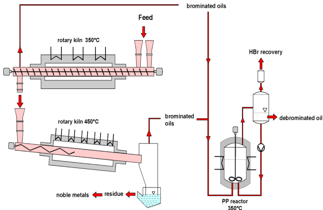
Schema F2 - Schema di principio del processo HALOCLEAN.
