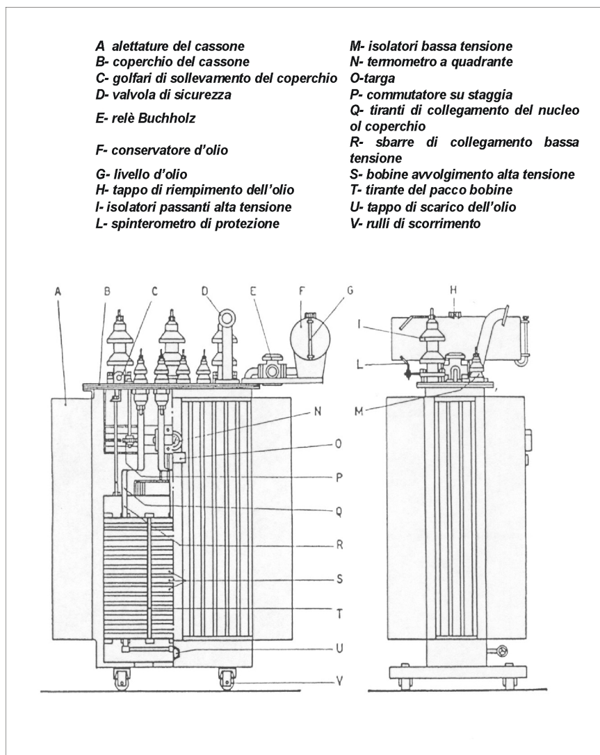
Figura C.1: Schema di un trasformatore - tipo distribuzione
