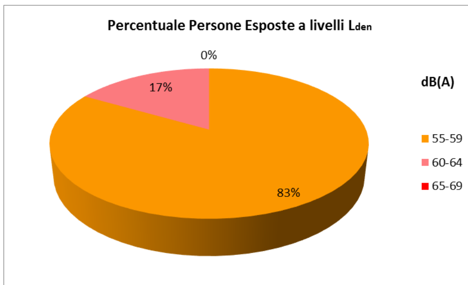
Figura 5.7 – Percentuale di persone esposte al rumore da traffico ferroviario – L_{den} per classe di esposizione
